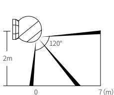
有效检测区域 (侧视图)
